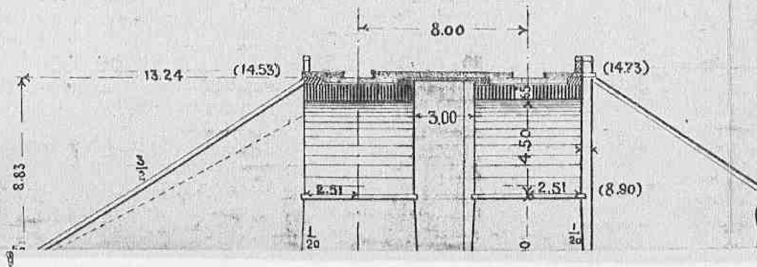
SEZIONE EF
